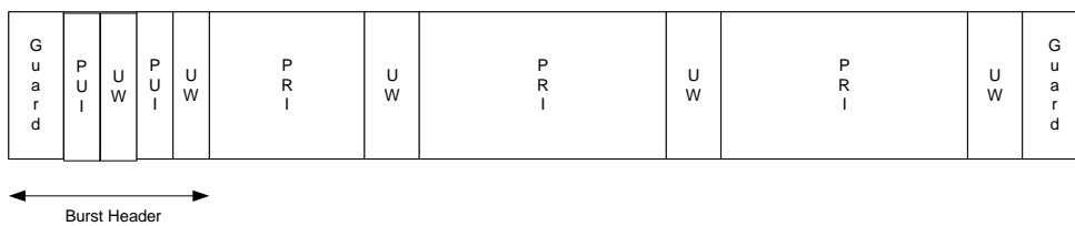
(d) PNB3(5,12) Downlink
