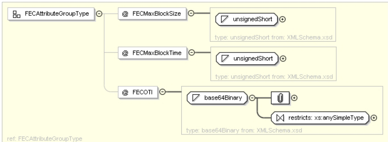
Figure 7ad: FECAttributeGroupType
