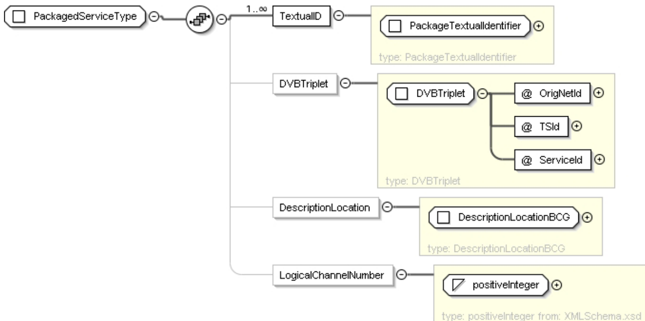
Figure 7az: PackagedServiceType
