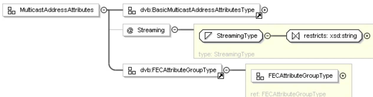
Figure 7ae: MulticastAddressAttribute
