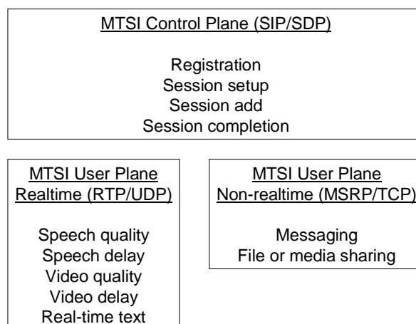
Figure 45: MTSI parameter structure
