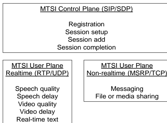
Figure 47: MTSI parameter structure
