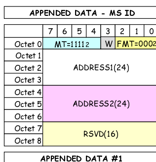
Figure 5.8: Appended_Data (MS ID)
