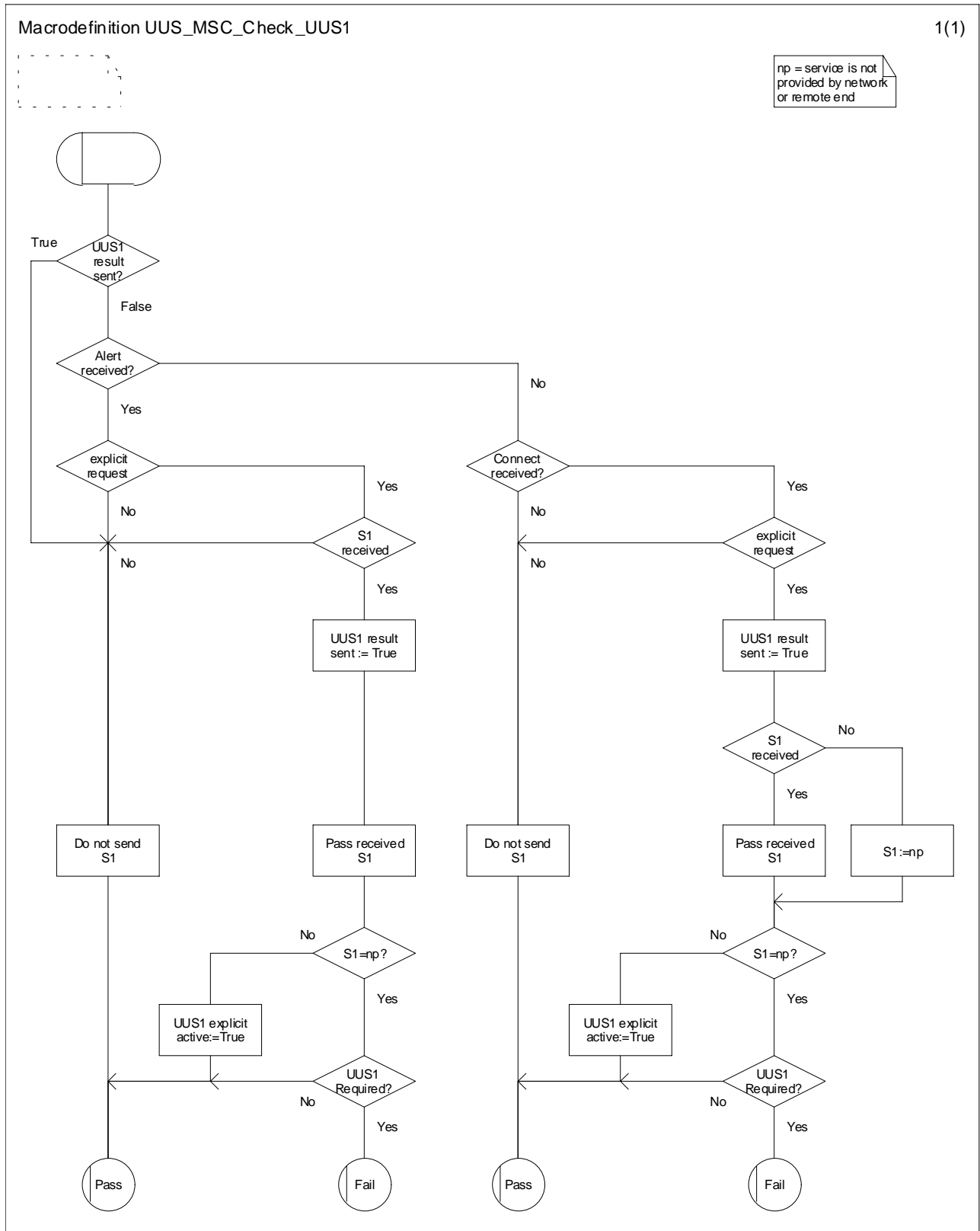
Figure 9.3.7: Macrodefinition UUS_MSC_Check_UUS1
