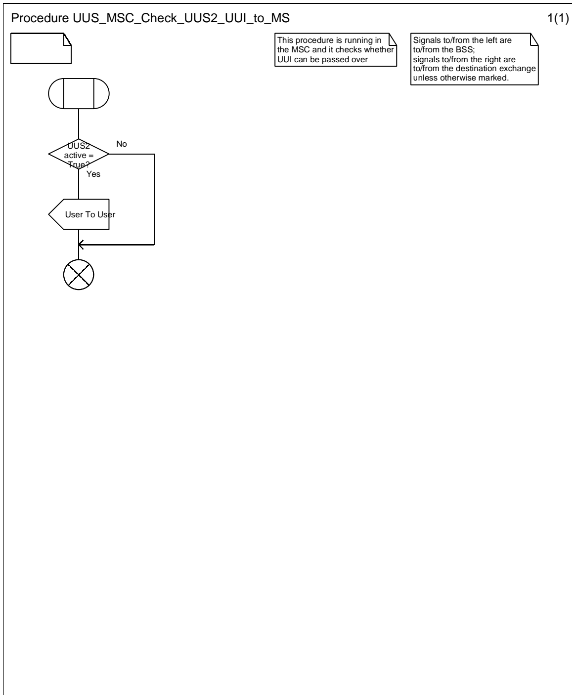
Figure 9.3.2: Procedure UUS_MSC_Check_UUS2_UUI_to_MS
