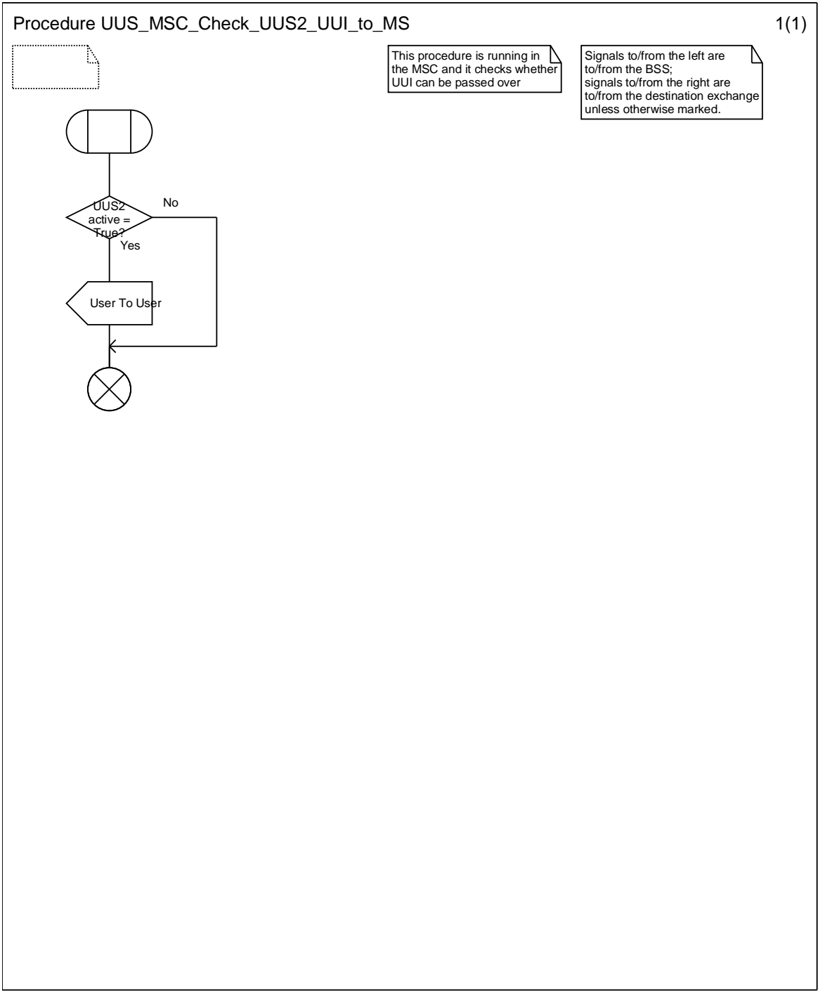
Figure 9.3.2: Procedure UUS_MSC_Check_UUS2_UUI_to_MS
