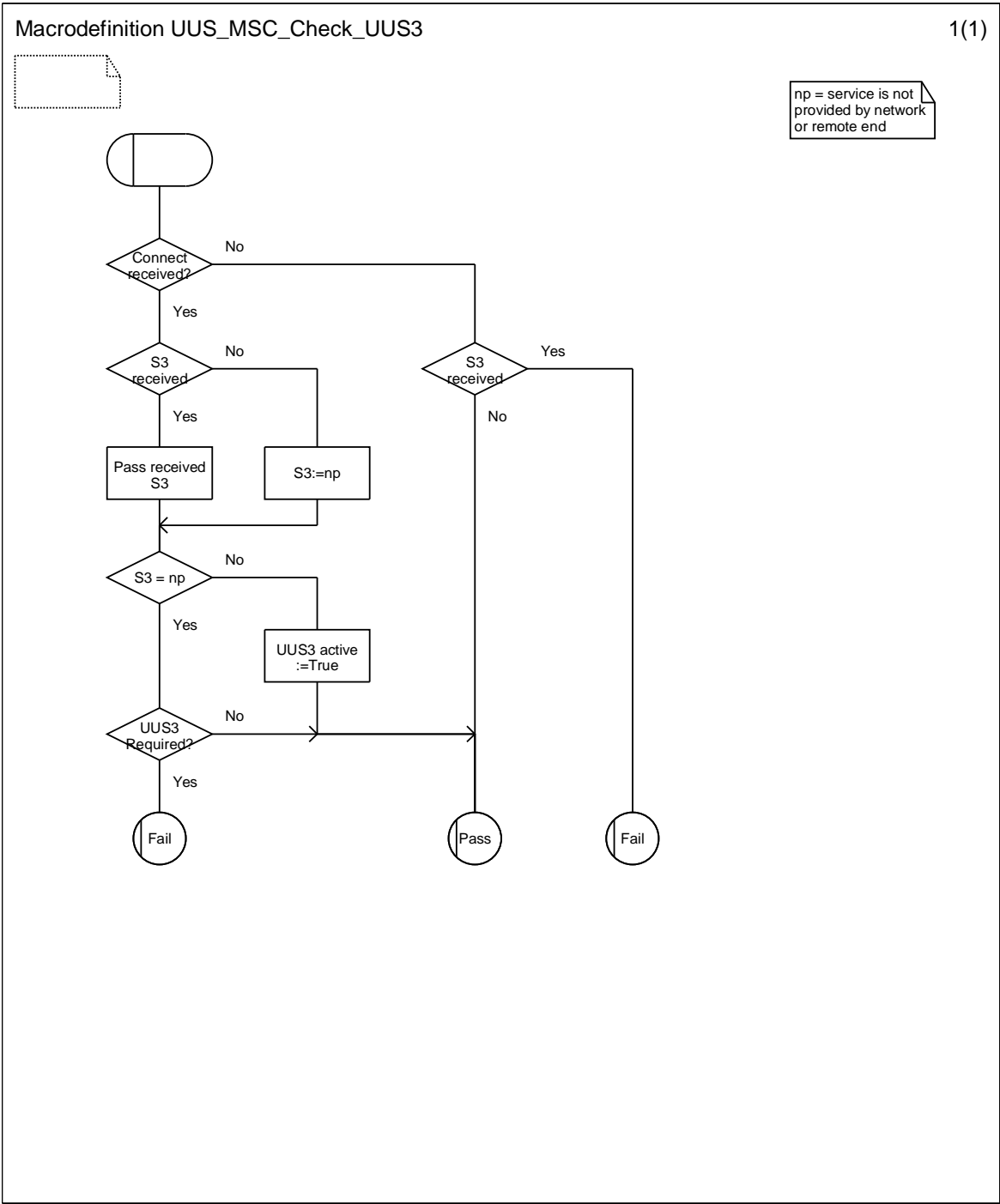
Figure 9.3.9: Macrodefinition UUS_MSC_Check_UUS3
