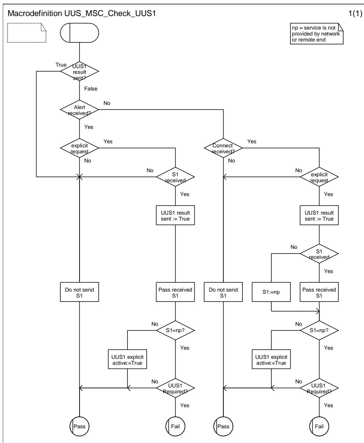
Figure 9.3.7: Macrodefinition UUS_MSC_Check_UUS1
