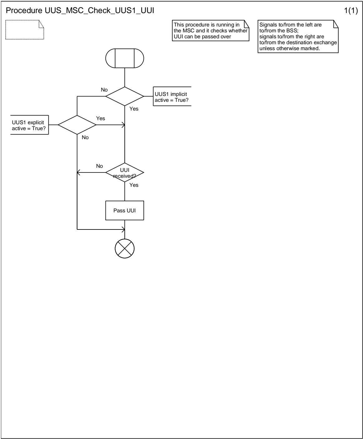
Figure 9.3.1: Procedure UUS_MSC_Check_UUS1_UUI
