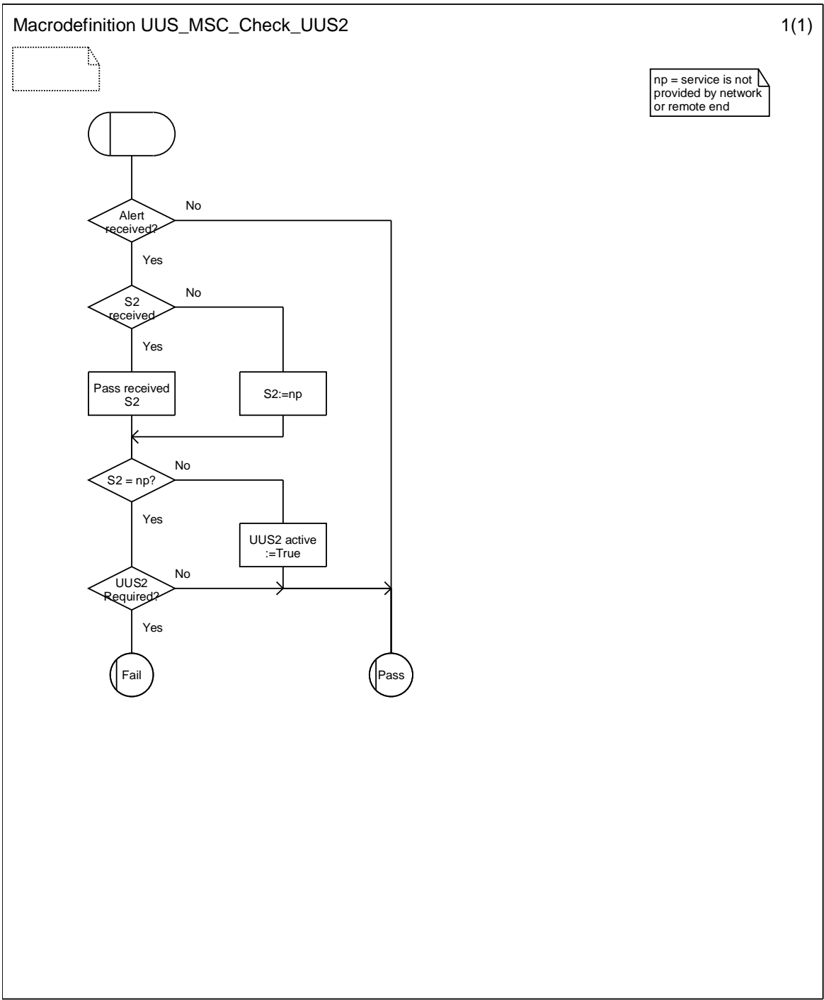
Figure 9.3.8: Macrodefinition UUS_MSC_Check_UUS2
