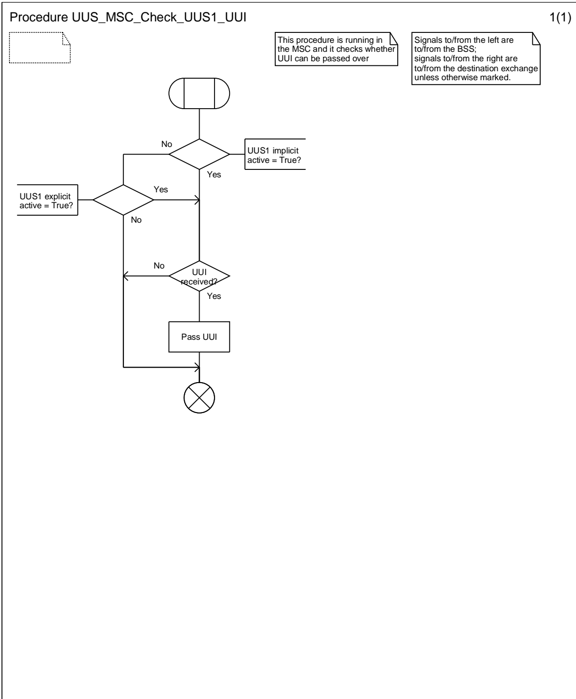
Figure 9.3.1: Procedure UUS_MSC_Check_UUS1_UUI
