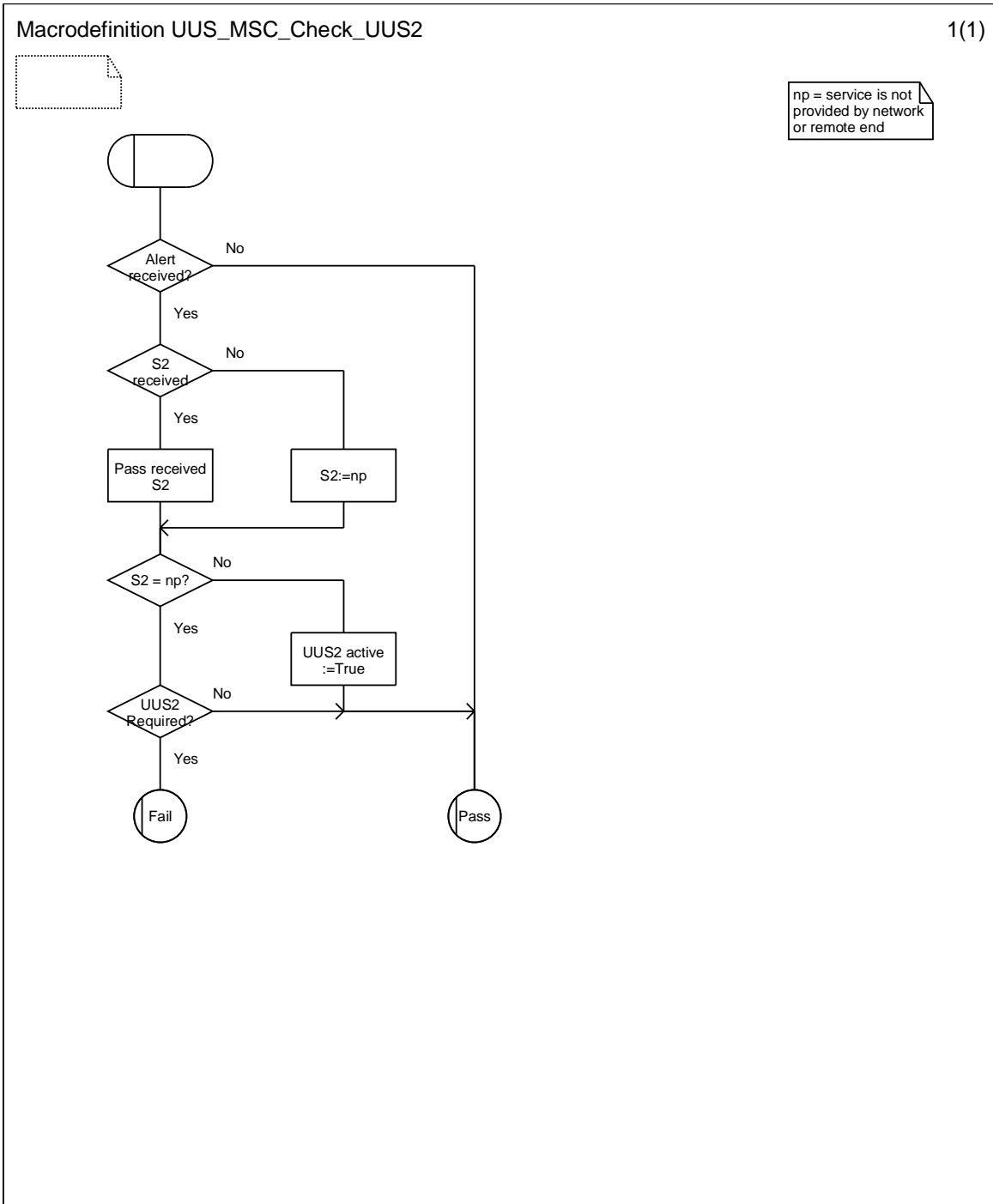
Figure 9.3.8: Macrodefinition UUS_MSC_Check_UUS2
