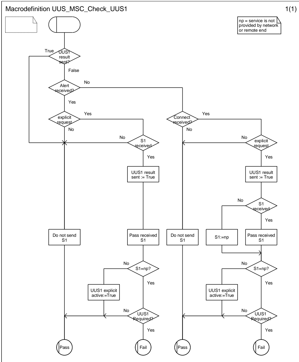
Figure 9.3.7: Macrodefinition UUS_MSC_Check_UUS1
