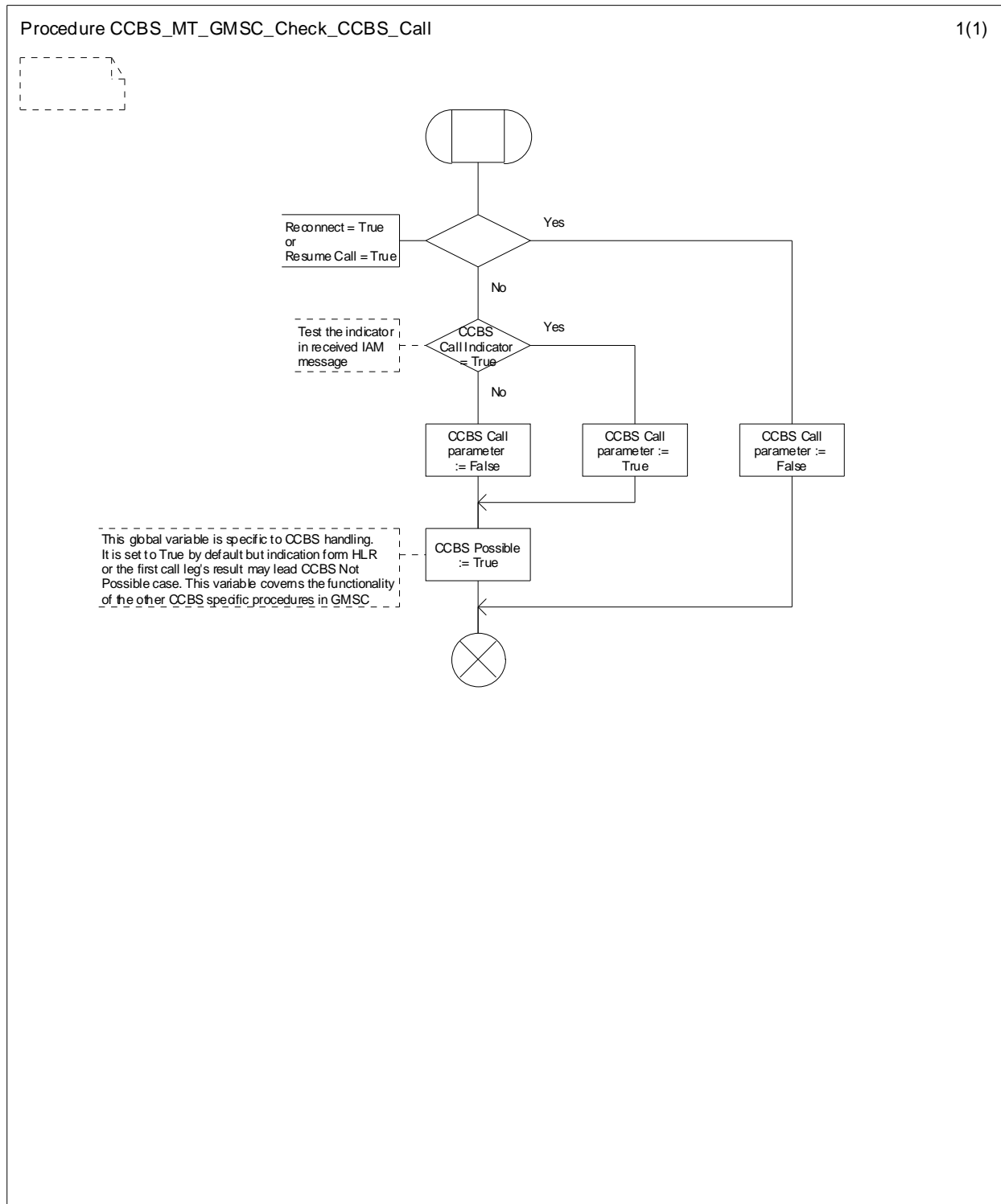
Figure 11.2.1.1: Procedure CCBS_MT_GMSC_Check_CCBS_Call
