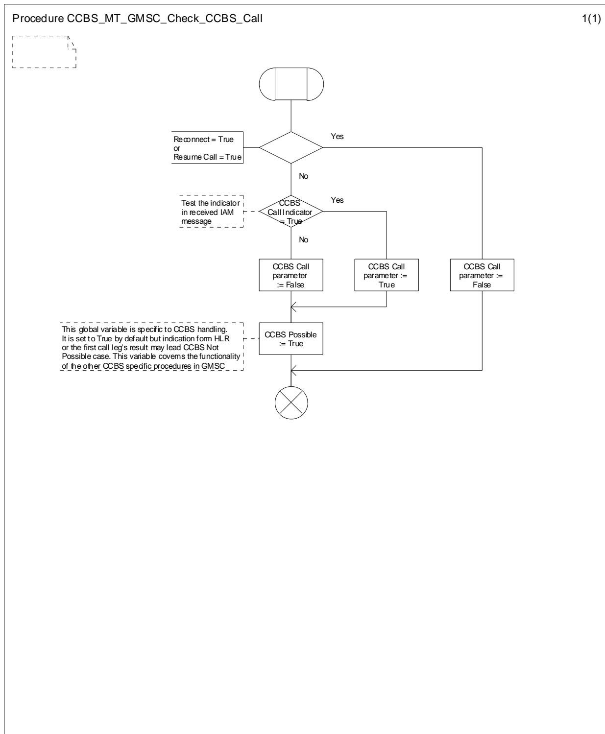
Figure 11.2.1.1: Procedure CCBS_MT_GMSC_Check_CCBS_Call
