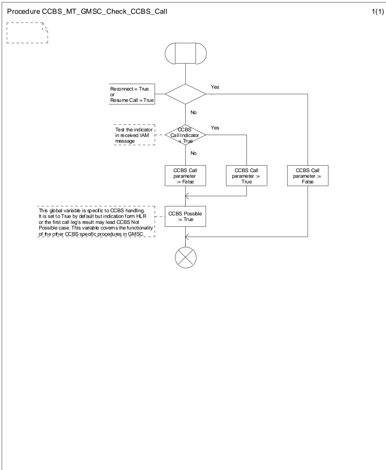
Figure 11.2.1.1: Procedure CCBS_MT_GMSC_Check_CCBS_Call
