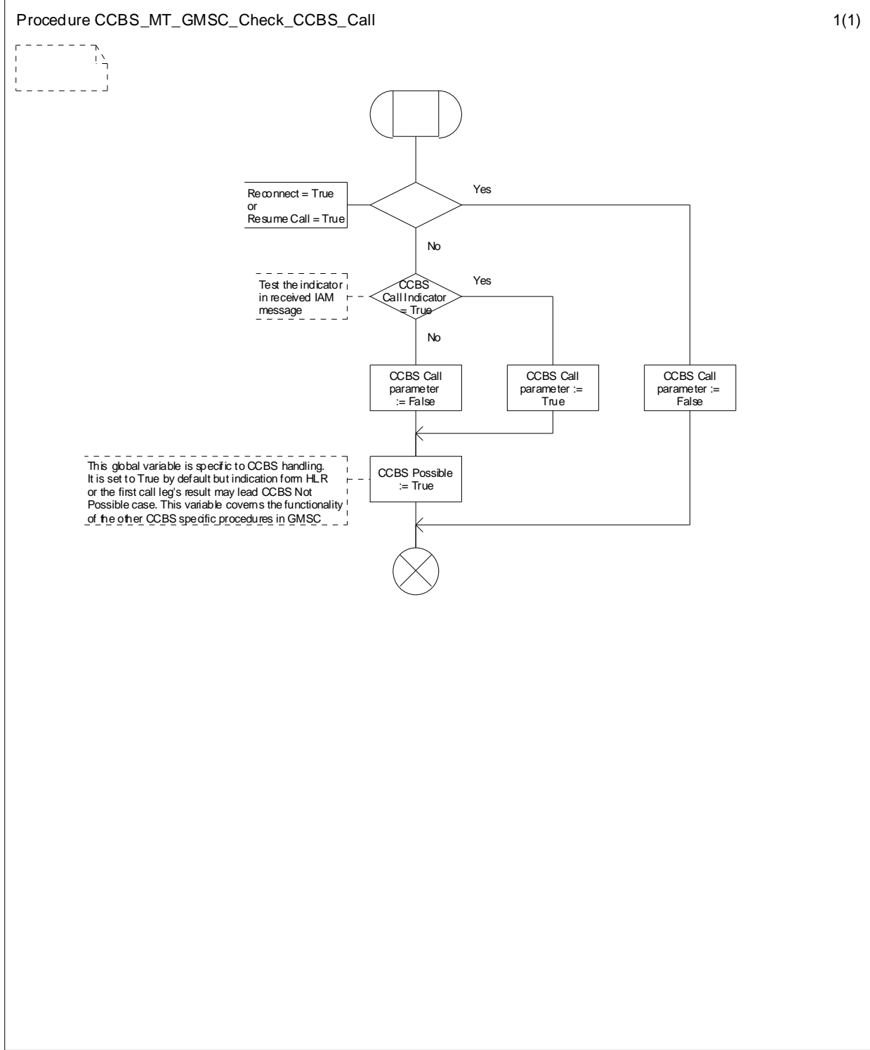
Figure 11.2.1.1: Procedure CCBS_MT_GMSC_Check_CCBS_Call
