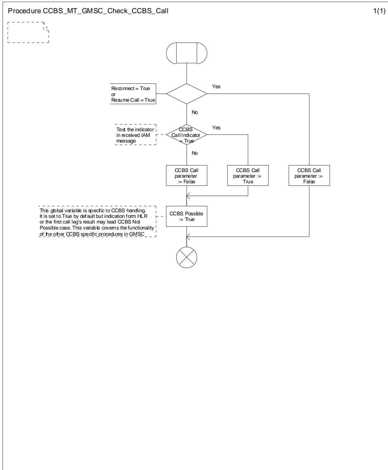
Figure 11.2.1.1: Procedure CCBS_MT_GMSC_Check_CCBS_Call
