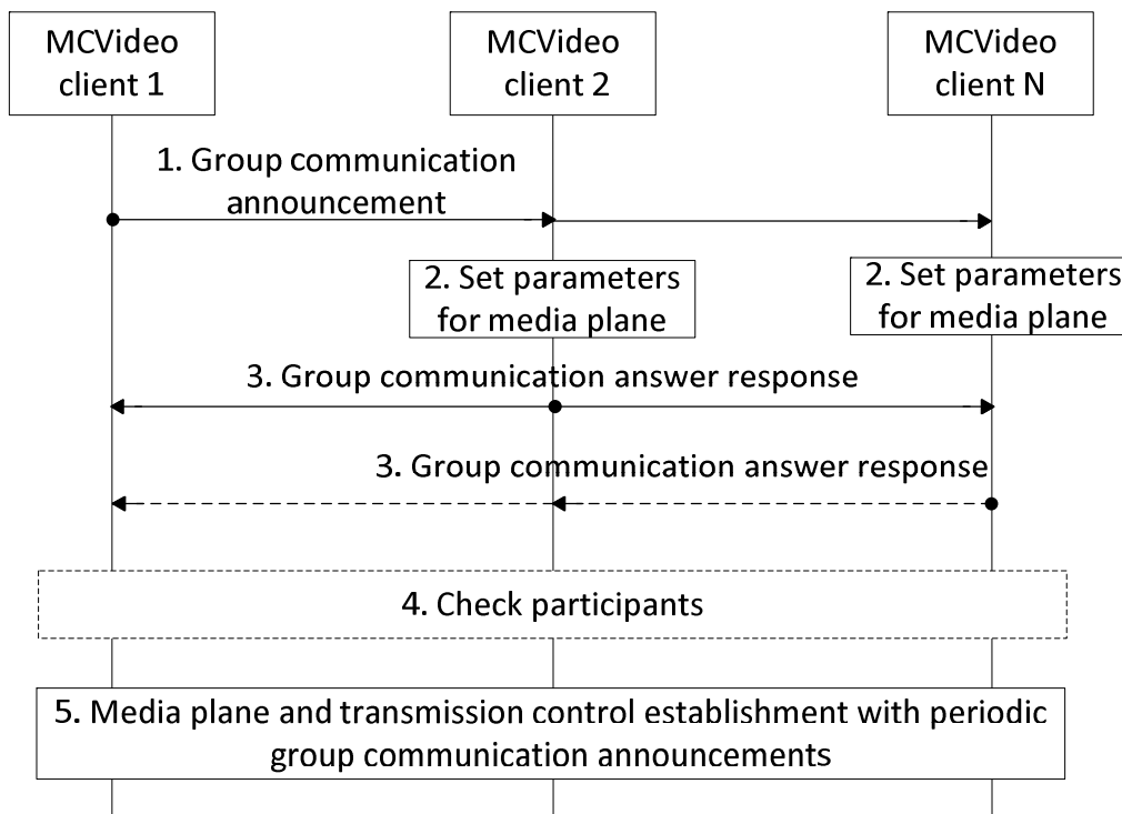
Figure 7.1.3.3.2-1: MCVidéo group communication setup
