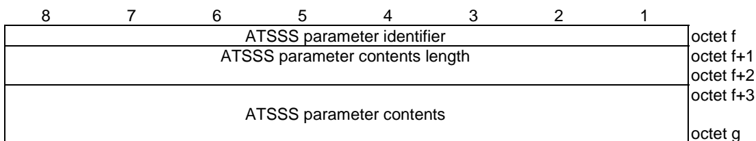
Figure 6.1.2-2: ATSSS parameter
