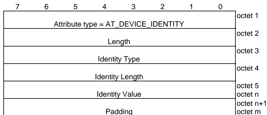
Figure 8.2.8.1-1: AT_DEVICE_IDENTITY attribute
