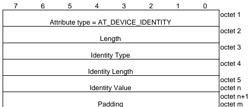
Figure 8.2.8.1-1: AT_DEVICE_IDENTITY attribute
