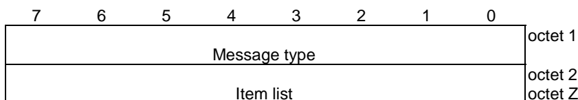
Figure 8.1.4.1-1: Message
