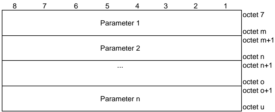
Figure 9.11.4.12.3: Parameters list
