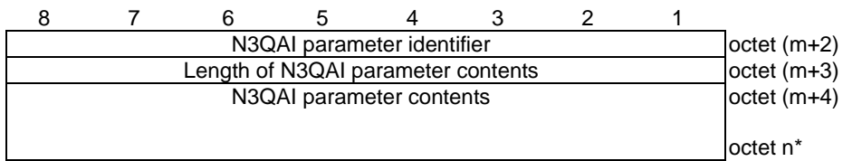
Figure 9.11.4.36.4: N3QAI parameter
