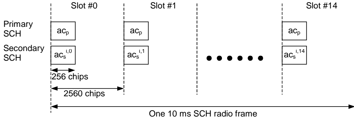
Figure x7: Structure of Synchronisation Channel (SCH)
