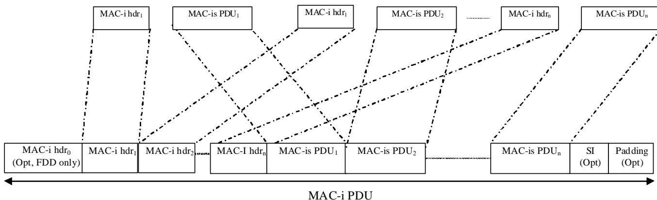
Figure 9.1.5.4a: MAC-i PDU.
