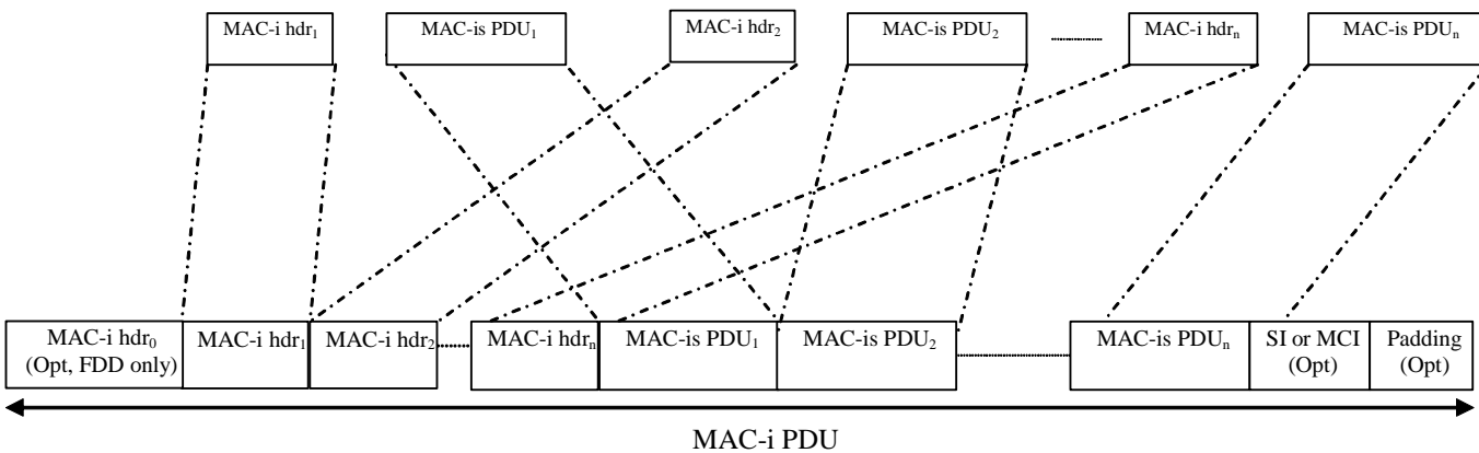
Figure 9.1.5-4a: MAC-i PDU.
