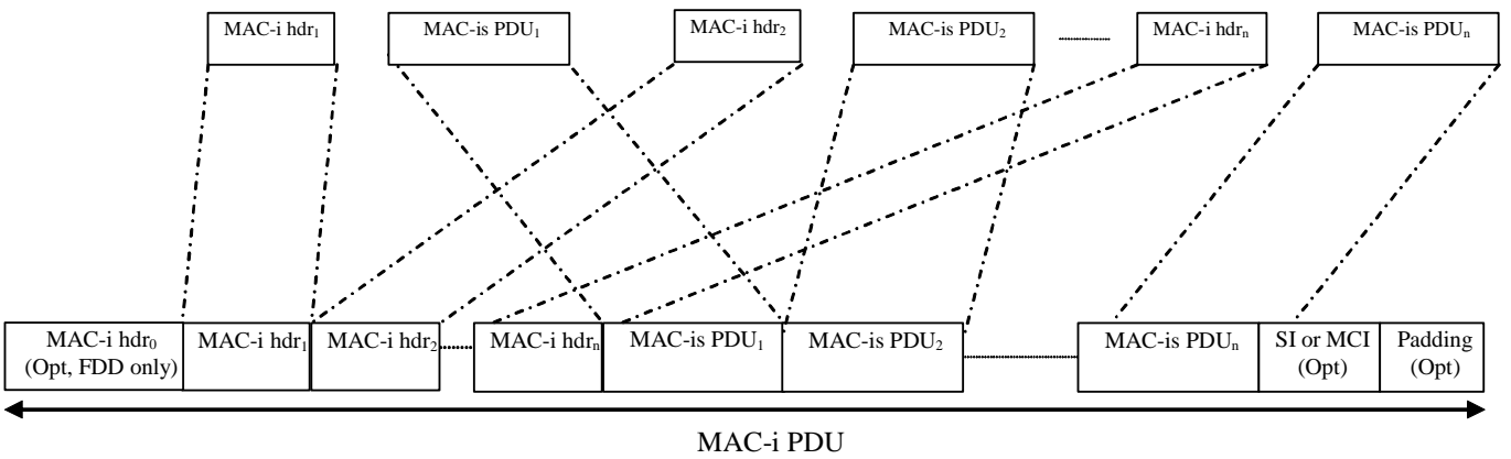
Figure 9.1.5-4a: MAC-i PDU.
