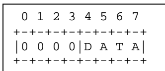
Figure 10.2a: Padding
