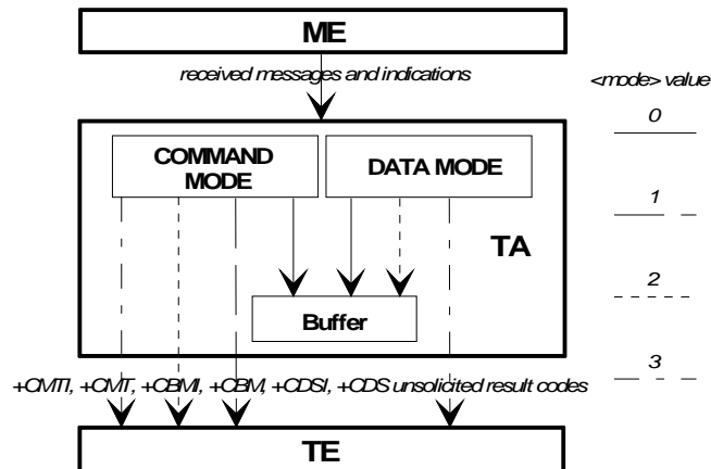
Figure 2: <mode> parameter
