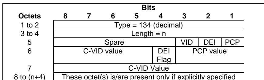
Figure 8.2.94-1: C-TAG (Customer-VLAN tag)
