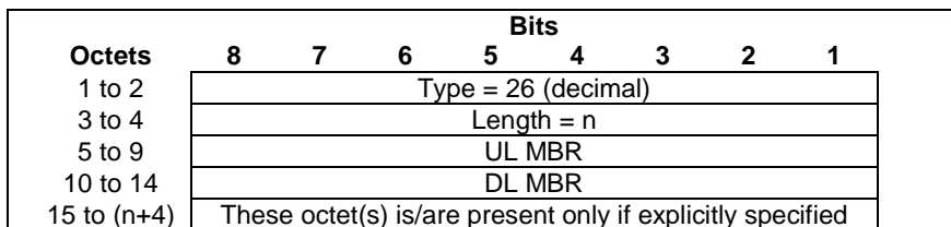
Figure 8.2.8-1: MBR
