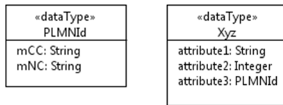
Figure 5.3.4.2-1: «dataType» notations
