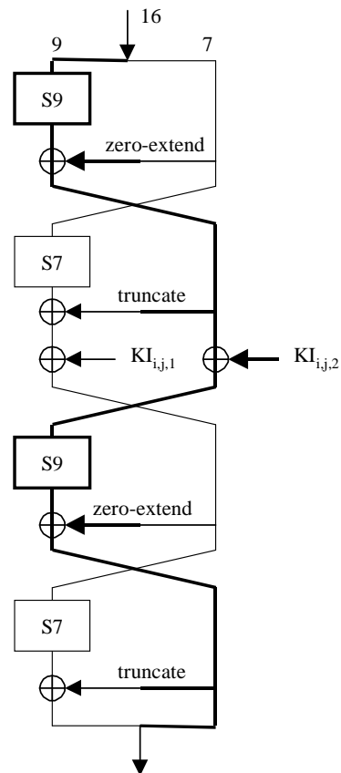
Fig.3: FI Function
