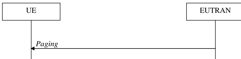
Figure 5.3.2.1-1: Paging
