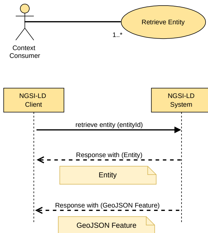
Figure 5.7.1.2-1: Retrieve Entity use case
