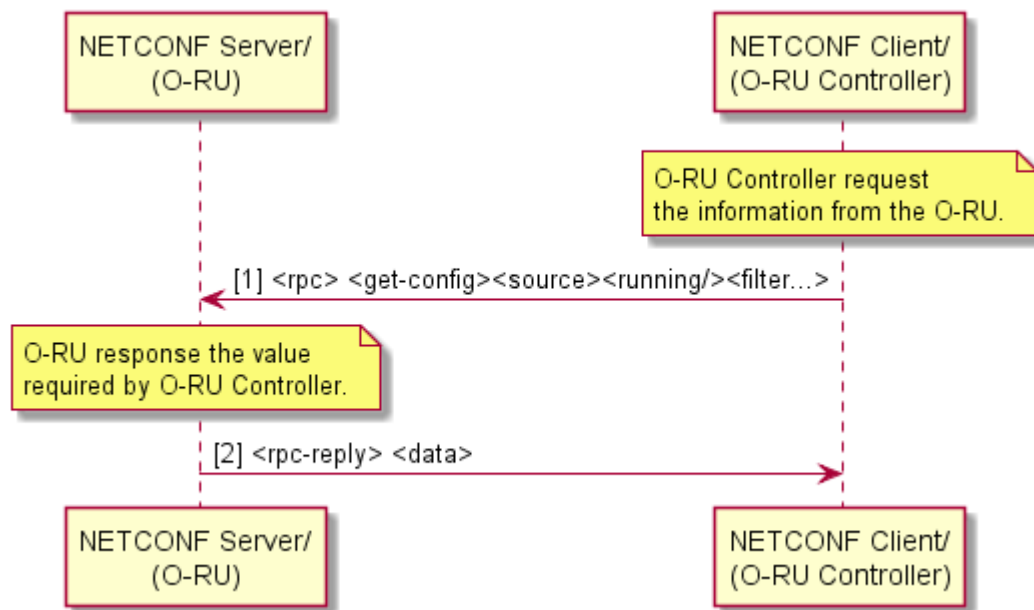
Figure 9.1.4-1: Retrieve Parameters
