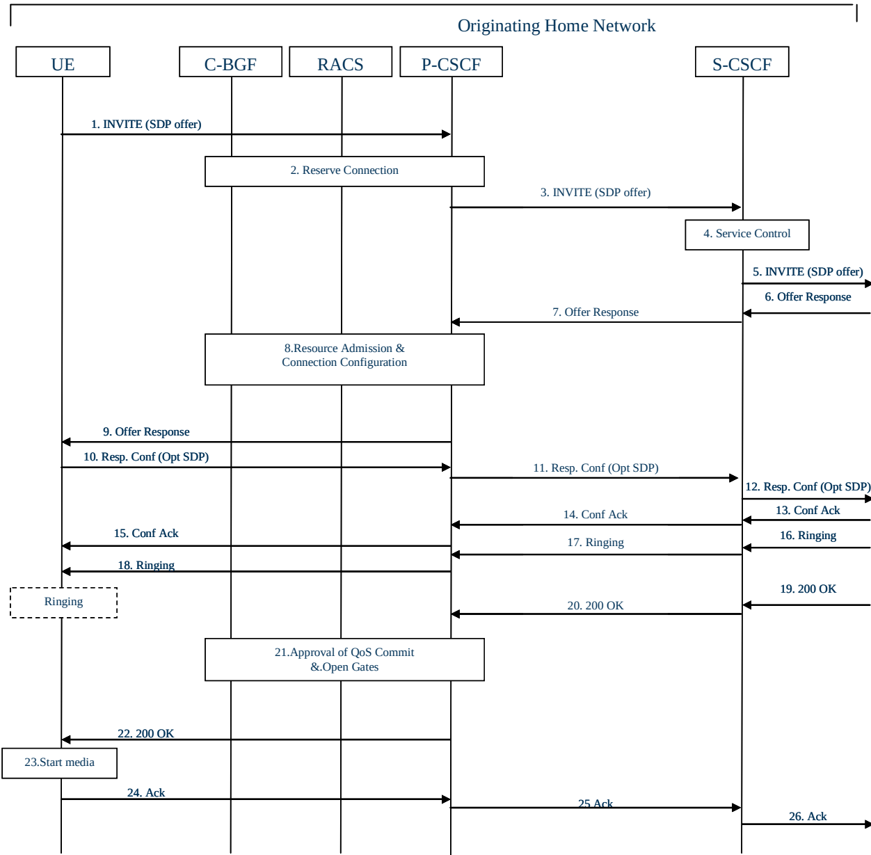
Figure N.1.1: Fixed xDSL originating - home (example flow)
