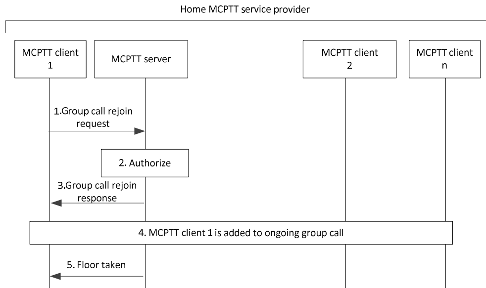
Figure 10.6.2.3.1.1.5-1: Rejoin call
