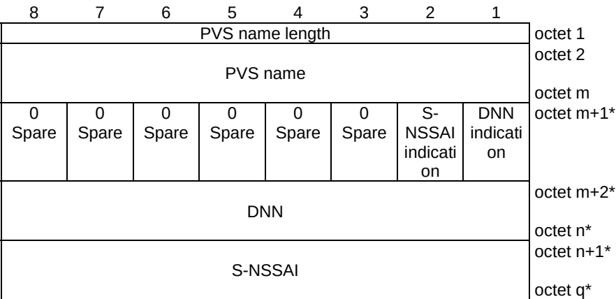
Figure 10.5.6.3.12-1/3GPP TS 24.008: PVS name
