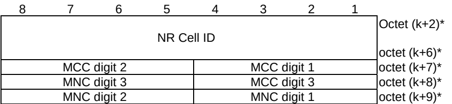
Figure 9.11.4.31.7: NR CGI
