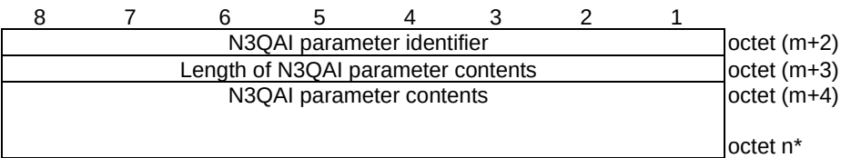
Figure 9.11.4.36.4: N3QAI parameter
