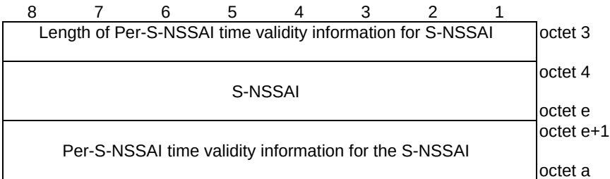
Figure 9.11.3.101.2: Per-S-NSSAI time validity information for S-NSSAI 1
