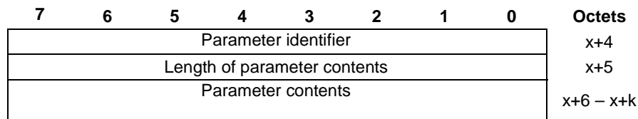
Figure 9.3.1.1-4: Parameter
