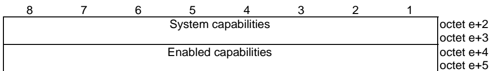
Figure 9.11.3: lldpRemSysCap
