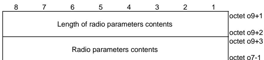
Figure 5.3.1.11: Radio parameters
