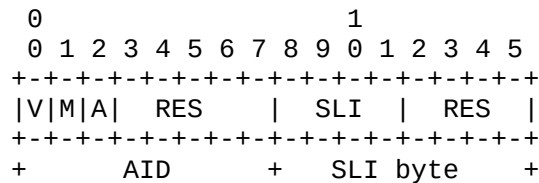
Figure A.3.5.7.4-1: DAS PI data byte
