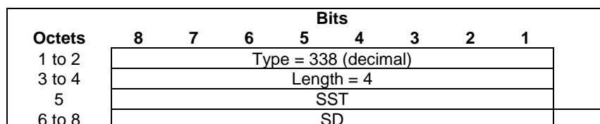
Figure 8.2.232-1: HPLMN S-NSSAI
