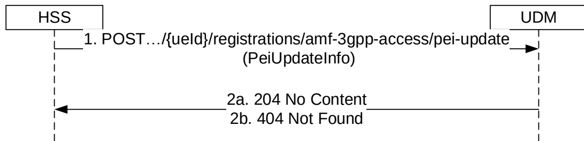
Figure 5.3.2.10.2-1: PEI Update
