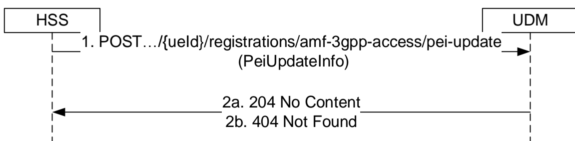
Figure 5.3.2.10.2-1: PEI Update
