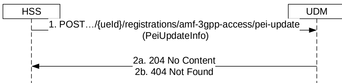
Figure 5.3.2.10.2-1: PEI Update
