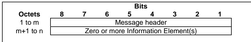
Figure 7.1.2.1-1: Message Format
