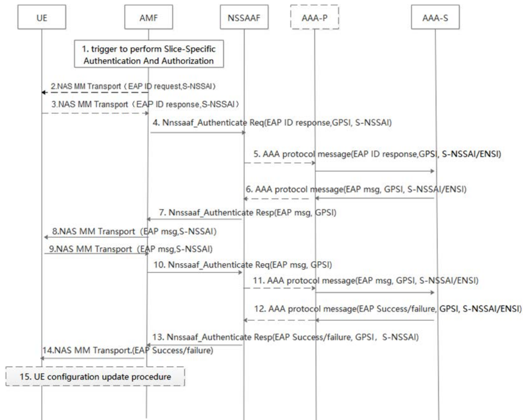
Figure 16.3-1: NSSAA procedure
