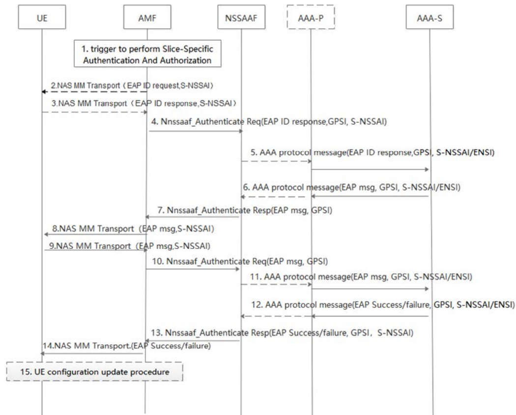
Figure 16.3-1: NSSAA procedure
